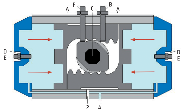
Grundstellung 0°
