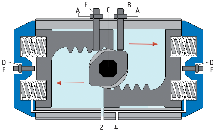
Schaltstellung 90°
