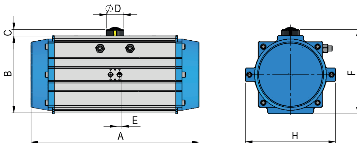
APD/APS-300 bis APD/APS-400
