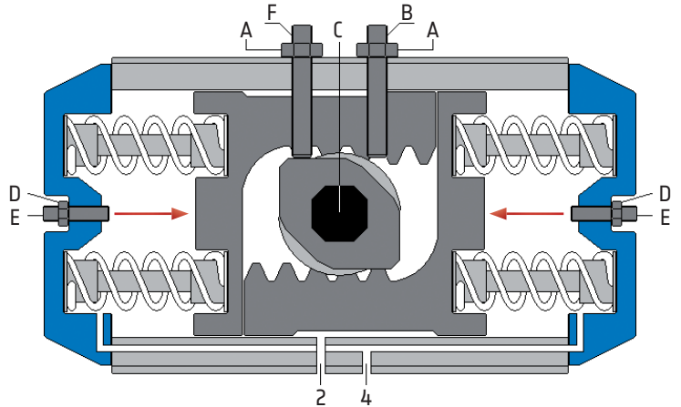
Grundstellung 0°
