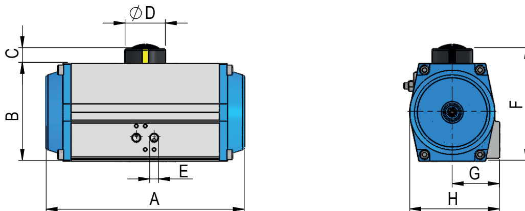
APD-040 bis APD/APS-270
