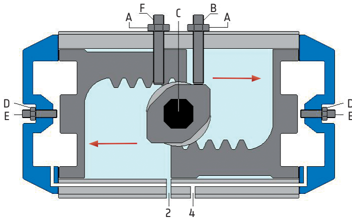
Schaltstellung 90°
